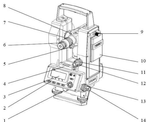
Рисунок 1- Устройство электронного теодолита
